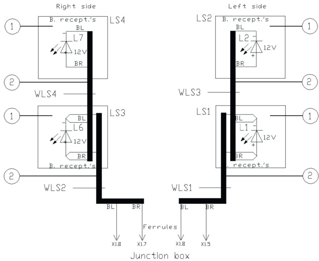
Elkretsschema sidomarkeringsljus
