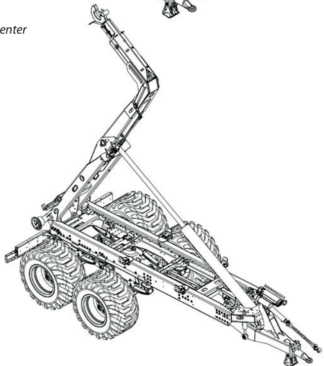
Tippningsläge B12
