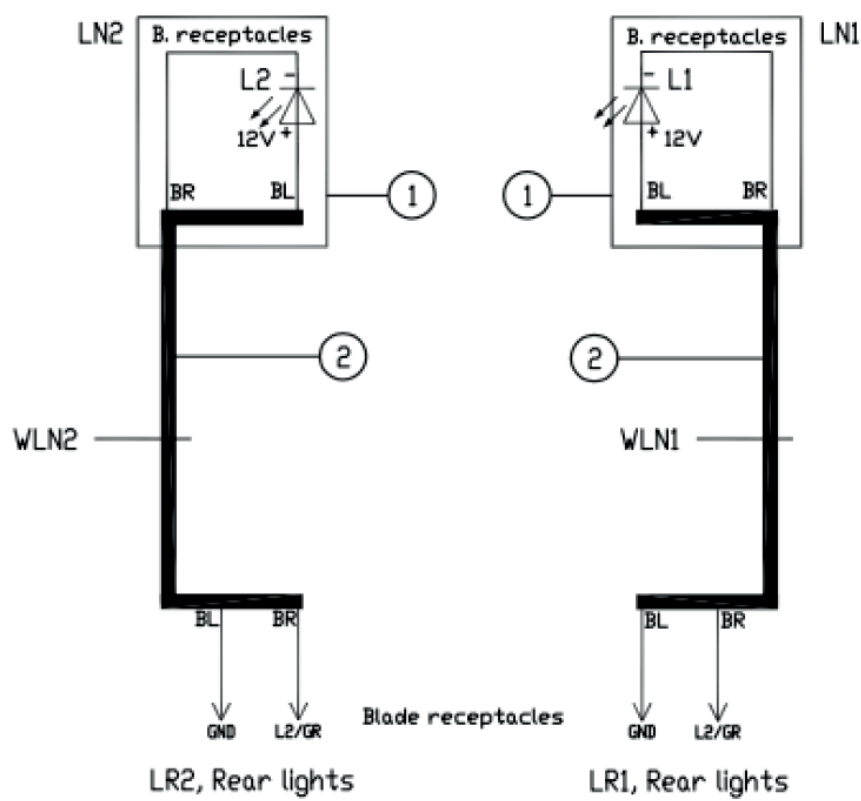
Elkretsschema registreringsskyltbelysning
