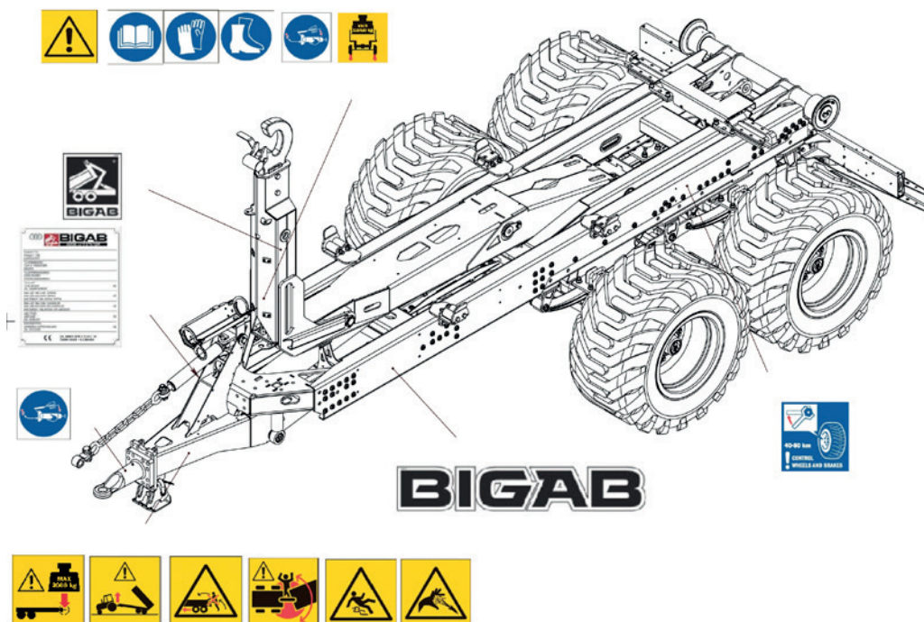
Dekalernas placering
