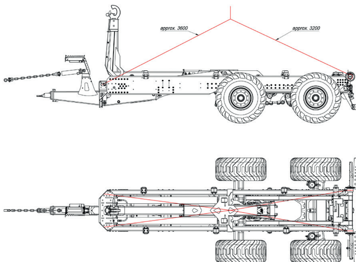
Løftepunkter for lasting/lossing
