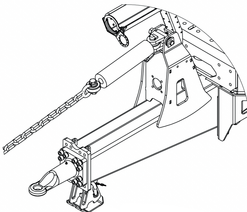
Parkeringsfot
