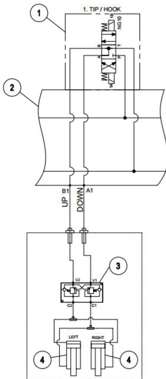
Kretsskjema hydraulikk
