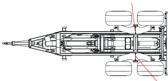
Jekkpunkter for mekanisk pendelboggi (boggiblokkering må være installert)
