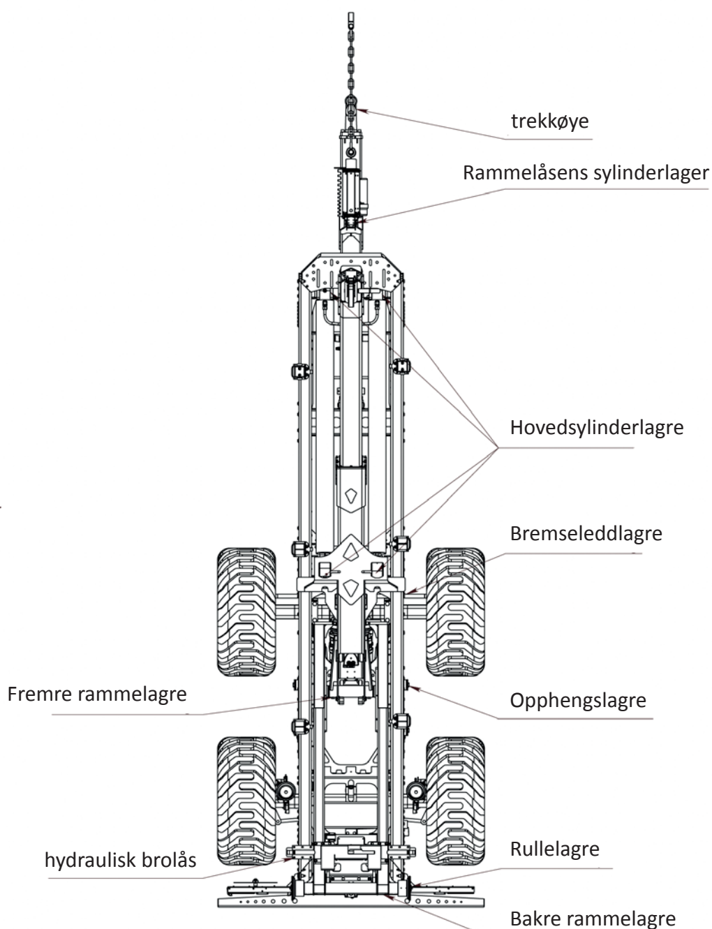
Figur 1. Smørepunkter på BIGAB
