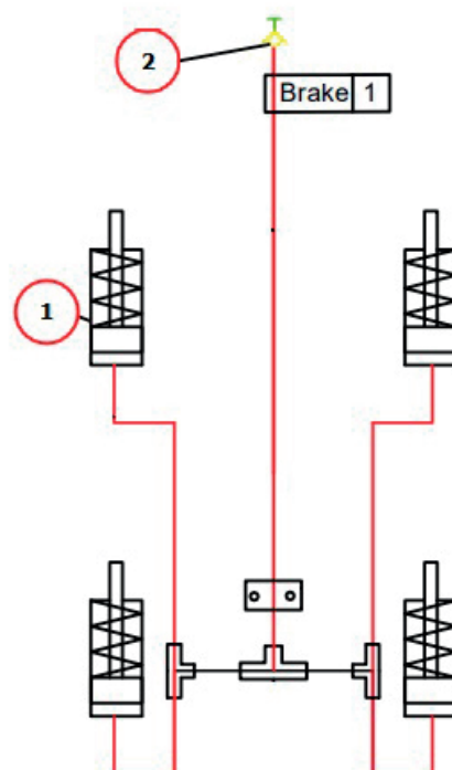
Kretsskjema bremser
