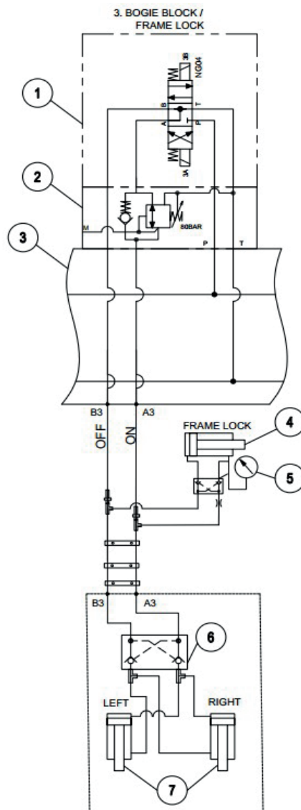
Boggiblokkering og rammelås
