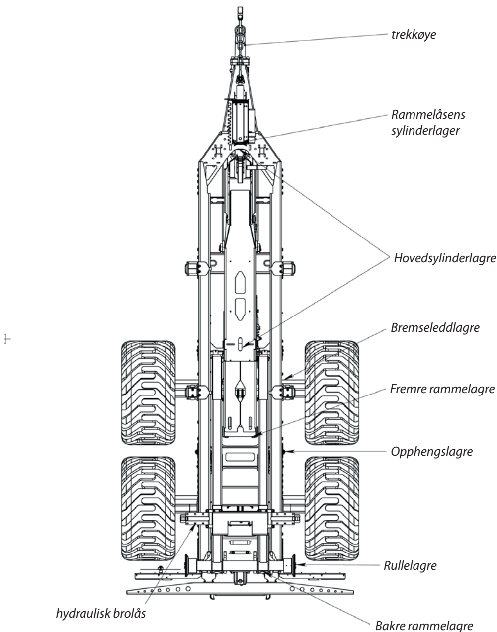
Figur 1. Smørepunkter på BIGAB
