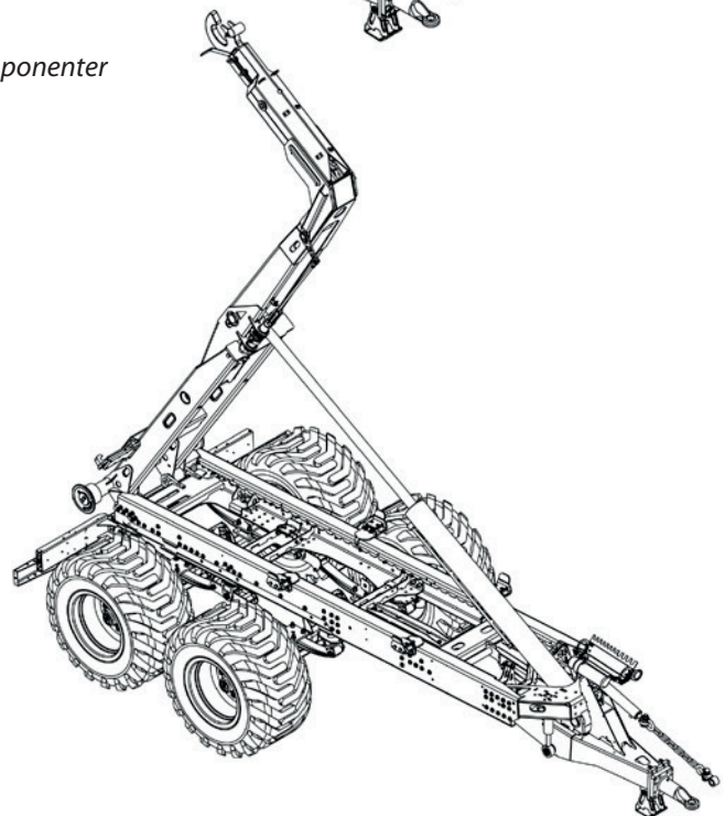
Tipping-posisjon 7-10
