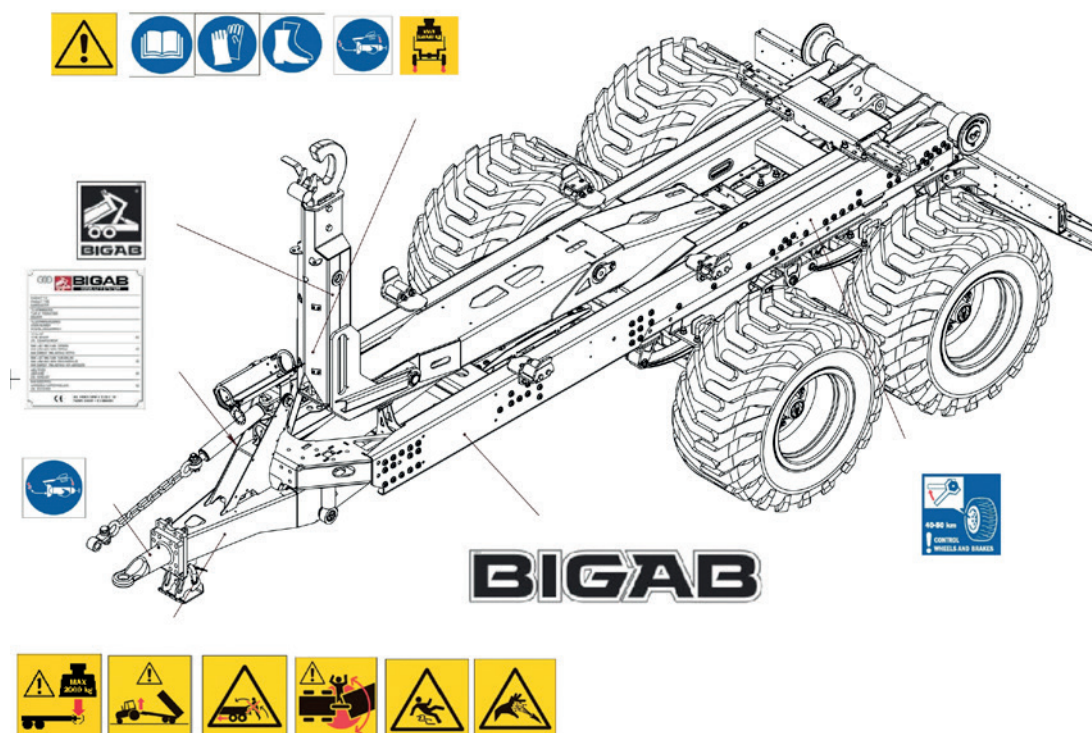
Plassering av etiketter på produktet
