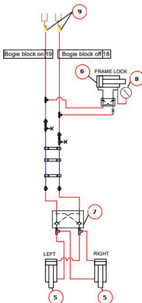
Boggiblokkering og rammelås
