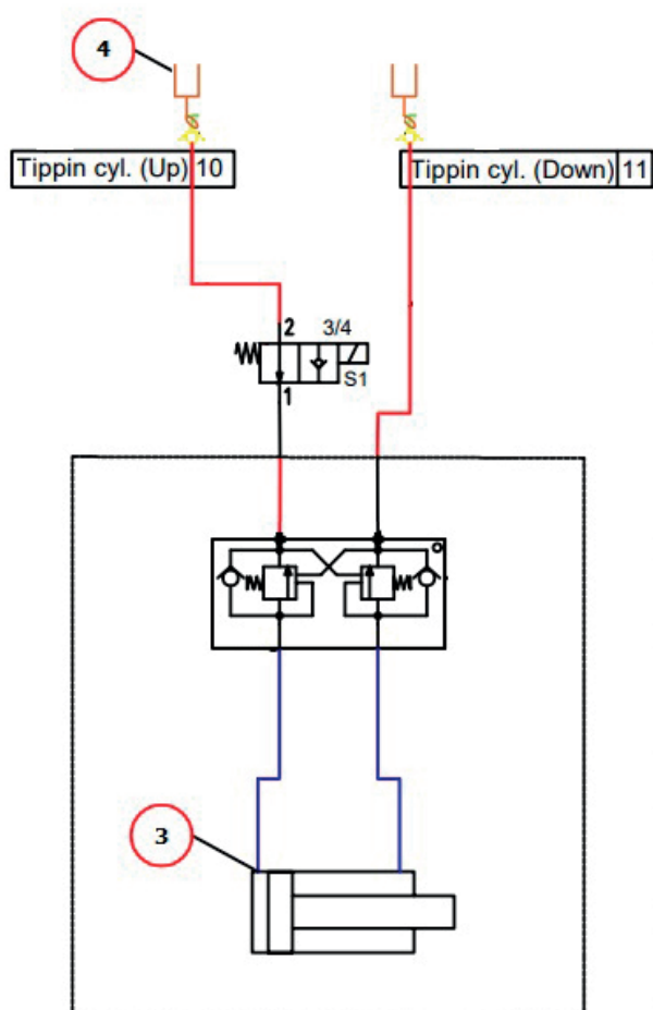
Kretsskjema hydraulikk
