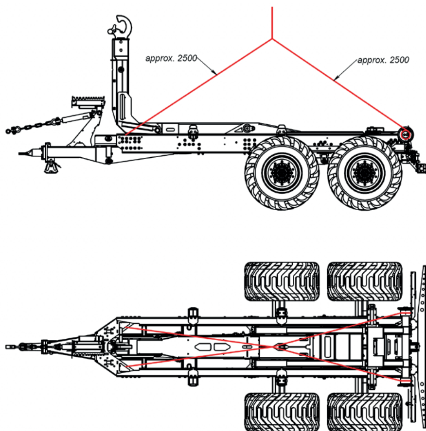
Løftepunkter for lasting/lossing
