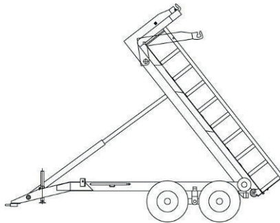
Angehobene Containerbrücke
