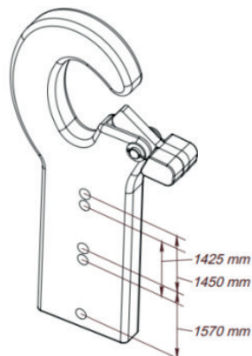
Haken
