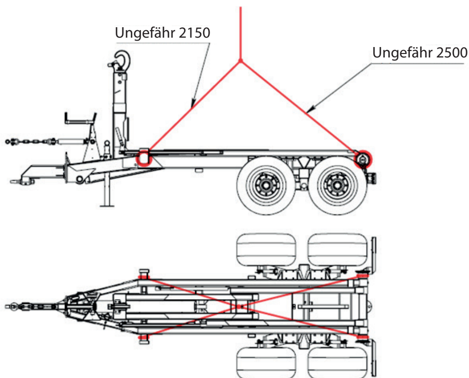
Hebepunkte zum Ab-/Aufladen
