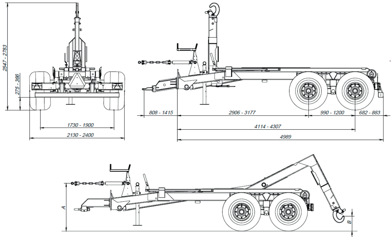
Maß von der Bodenfläche bis zur Rahmensicherung (A)
