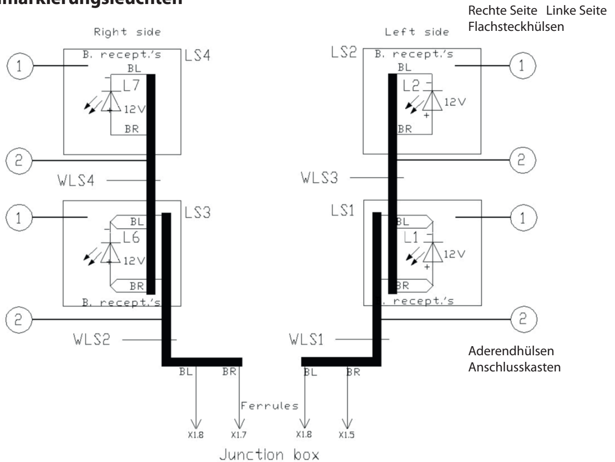
Schaltplan für Seitenmarkierungsleuchten
