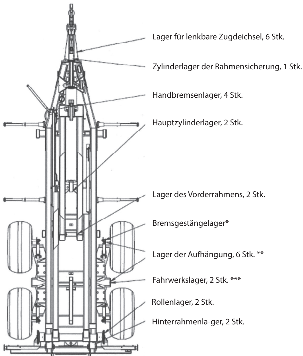
Abbildung 1. Schmierpunkte des BIGAB
