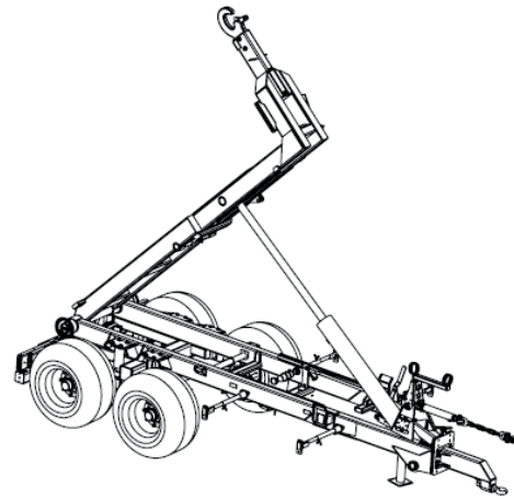
Kippposition 8-12, 10-14, 12-15 und 14-17
