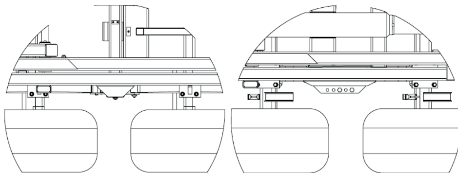
Festziehen der Bolzen beim BIGAB Tandem-Parabelfahrwerk Festziehen der Bolzen beim BIGAB gefederten Pendelfahrwerk
