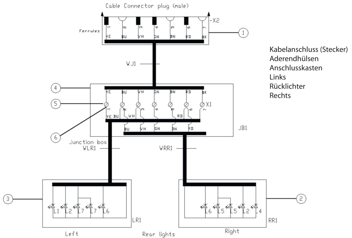
Schaltplan Rücklichter
