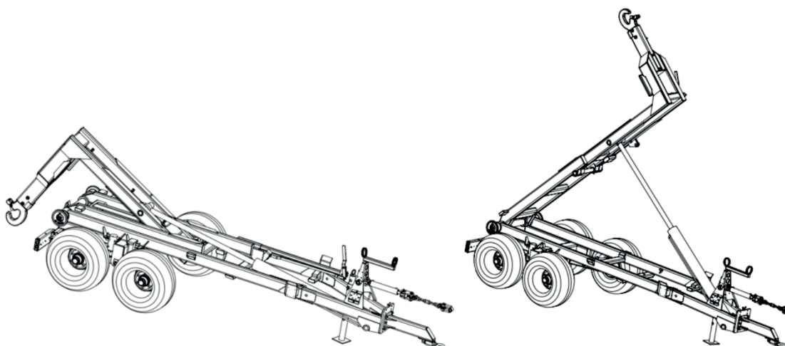
Auf-/Abrollposition 7-10
