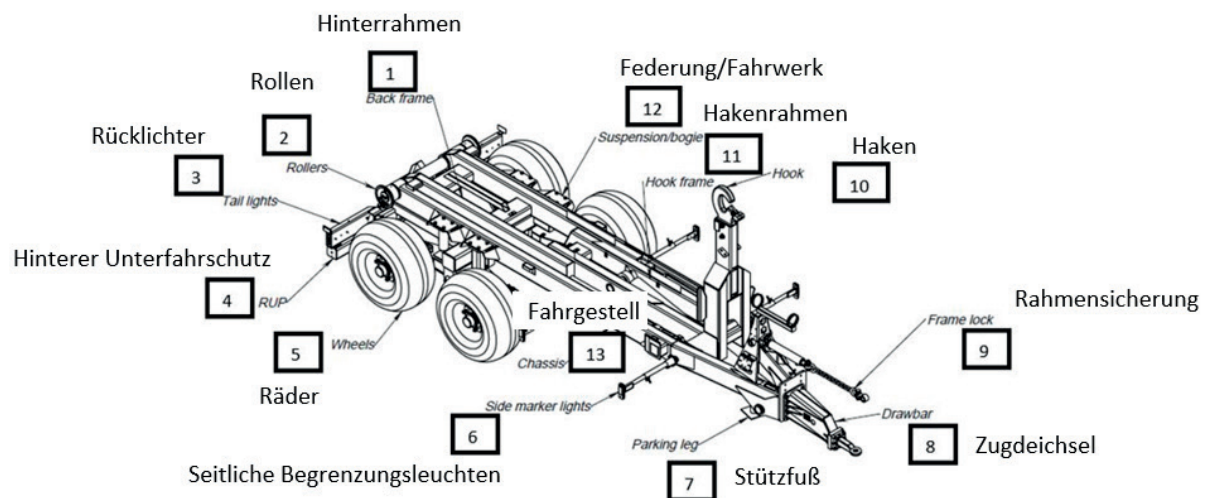
Hauptkomponenten des Anhängers
