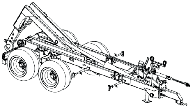
Auf-/Abrollposition 8-12, 10-14, 12-15 und 14-17
